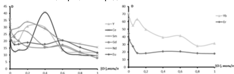
Рисунок 5 - Зависимость коэффициентов распределения РЗМ от хлорид аниона при экстракции нафтенной кислотой в о-ксилоле, в соотношении фаз 1 к 10 и кислотности водной фазы 5 \pm 0,1 единиц рН, для: а) легких лантаноидов и иттрия; б) для тяжелых лантаноидов
